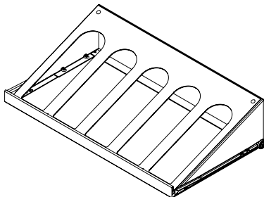
Figure 32 étagère-présentoir pour 5 bouteilles avec tapis atténuateur de vibrations
