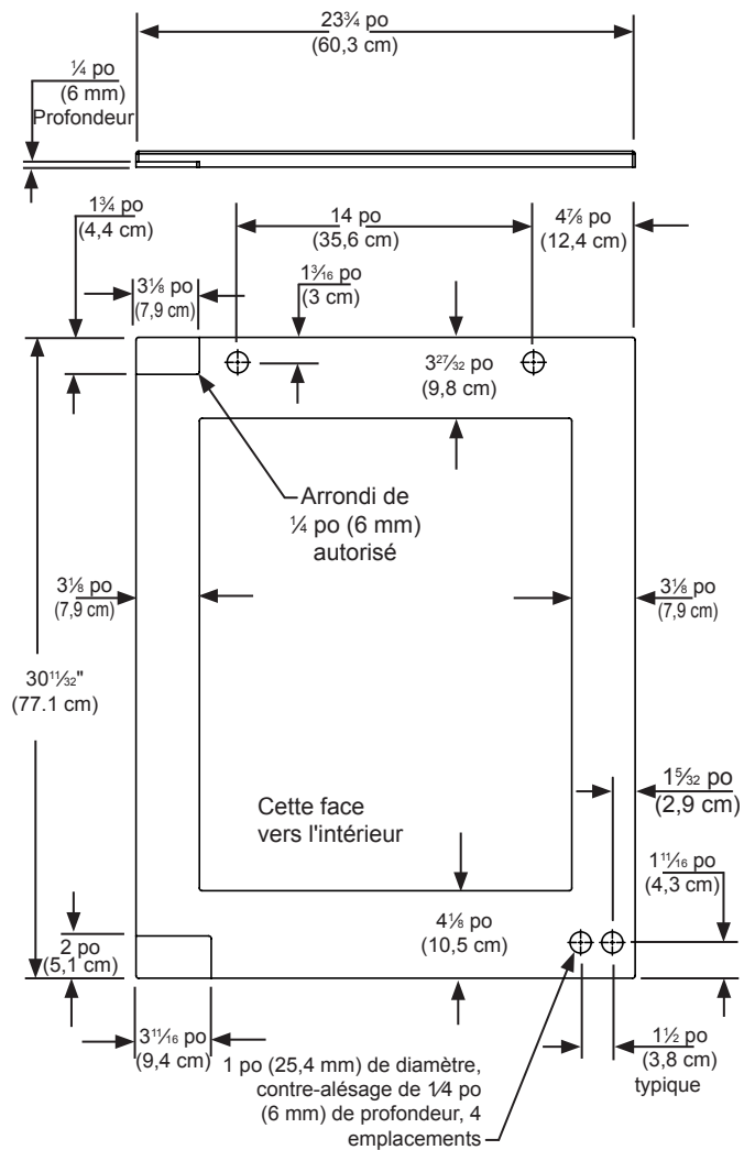
Figure 21 Porte à charnières à droite Appareil de largeur 24 po (61 cm)
